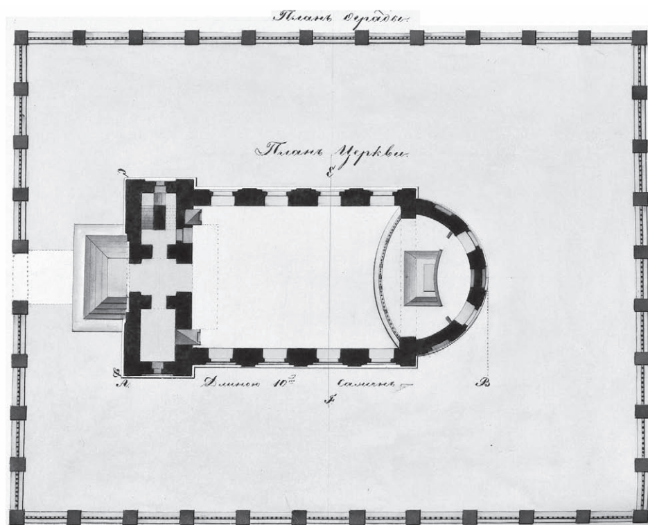
План костёла в г. Оренбурге. Проект 1844 г.
