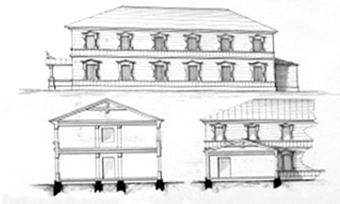
Проект 2-этажного келейного корпуса обители. 1893 г.
