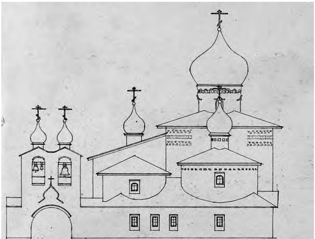
Проект Нарвского подворья Илецкого Николаевского монастыря
