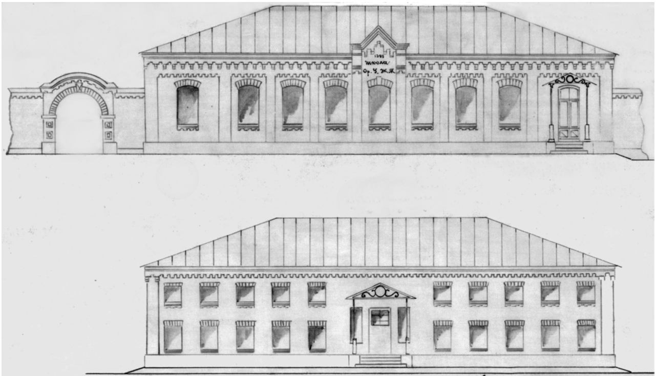
Проект нового здания церковно-приходской школы при Оренбургском Успенском женском монастыре. 1899 г.
