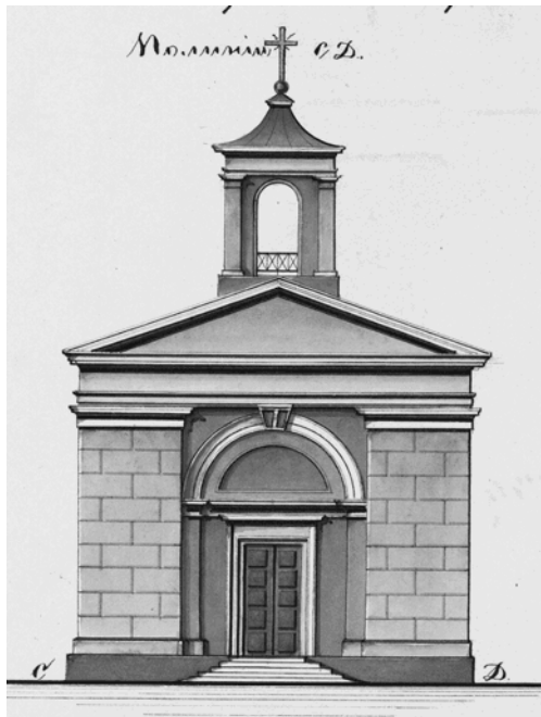
Передний фасад костёла в г. Оренбурге. Проект 1844 г.
