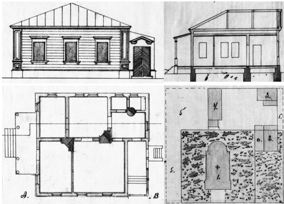
Проект расширения дома католического священника в Оренбурге. 1889 г.
