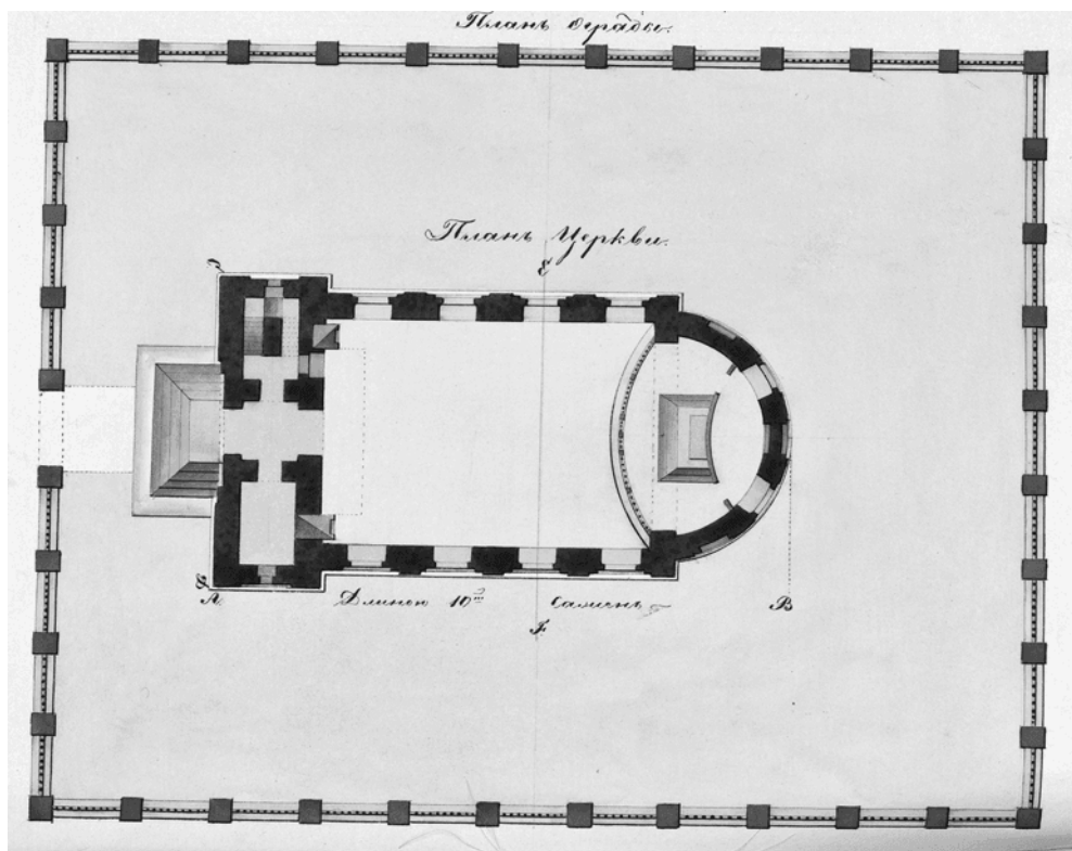
План костёла в г. Оренбурге. Проект 1844 г.
